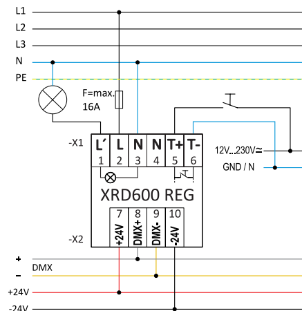
Blackschaltbild
