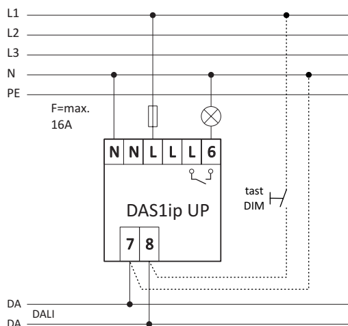
Anschlussbild
